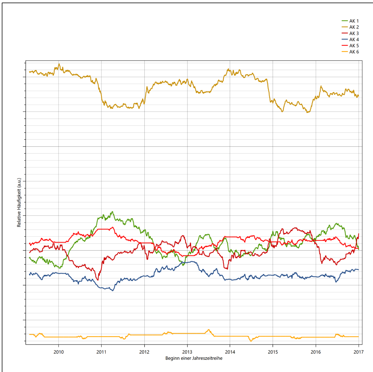
Abbildung 14: Prüfung auf vollständige und homogene Daten der modellierten Daten anhand der Verteilung der Ausbreitungsklasse
