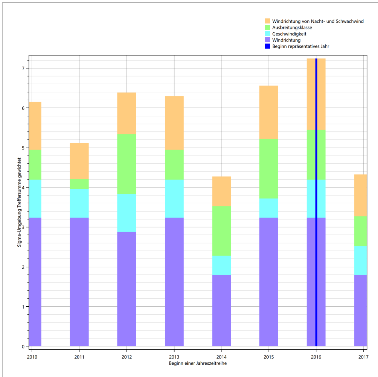
Abbildung 16: Gewichtete \sigma -Umgebung-Treffersumme und Einzelwerte als Maß für die Ähnlichkeit der einzelnen Testzeiträume zu je einem Jahr (Jahreszeitreihe) mit dem Gesamtzeitraum
