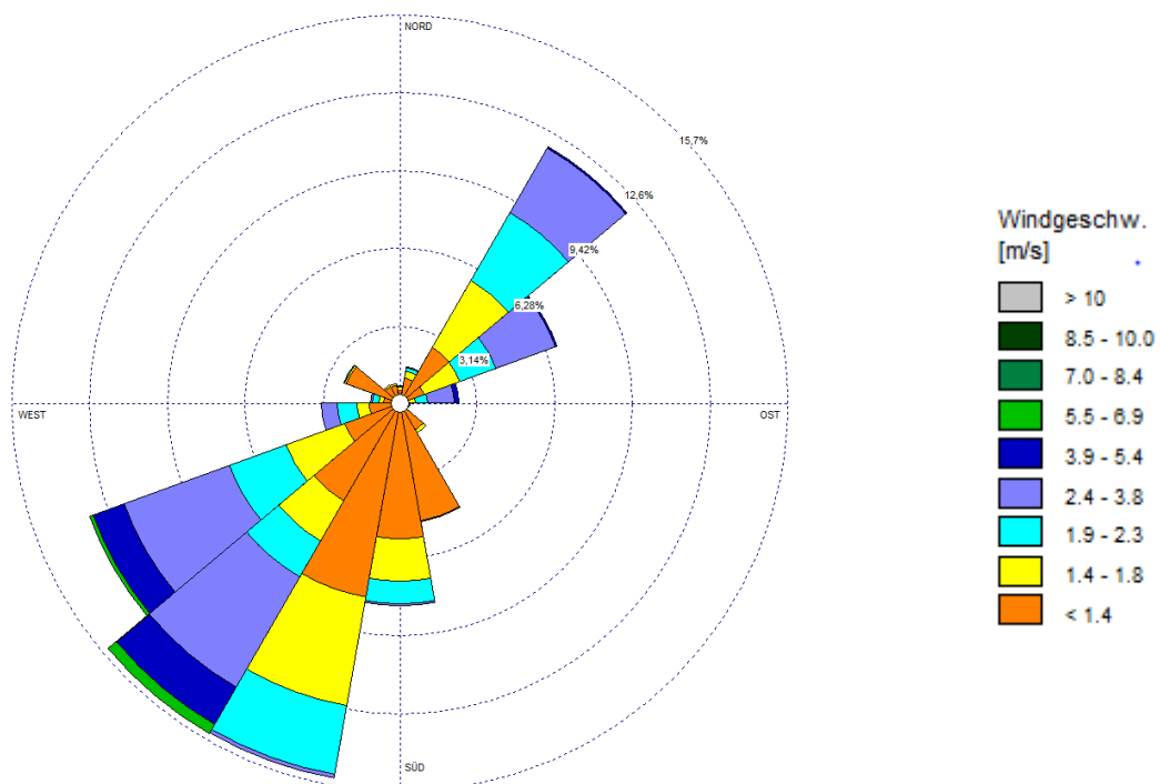
Abbildung 7: Windrichtungs- und Windgeschwindigkeitsverteilung des verwendeten meteorologischen Datensatzes (synAkterm)
