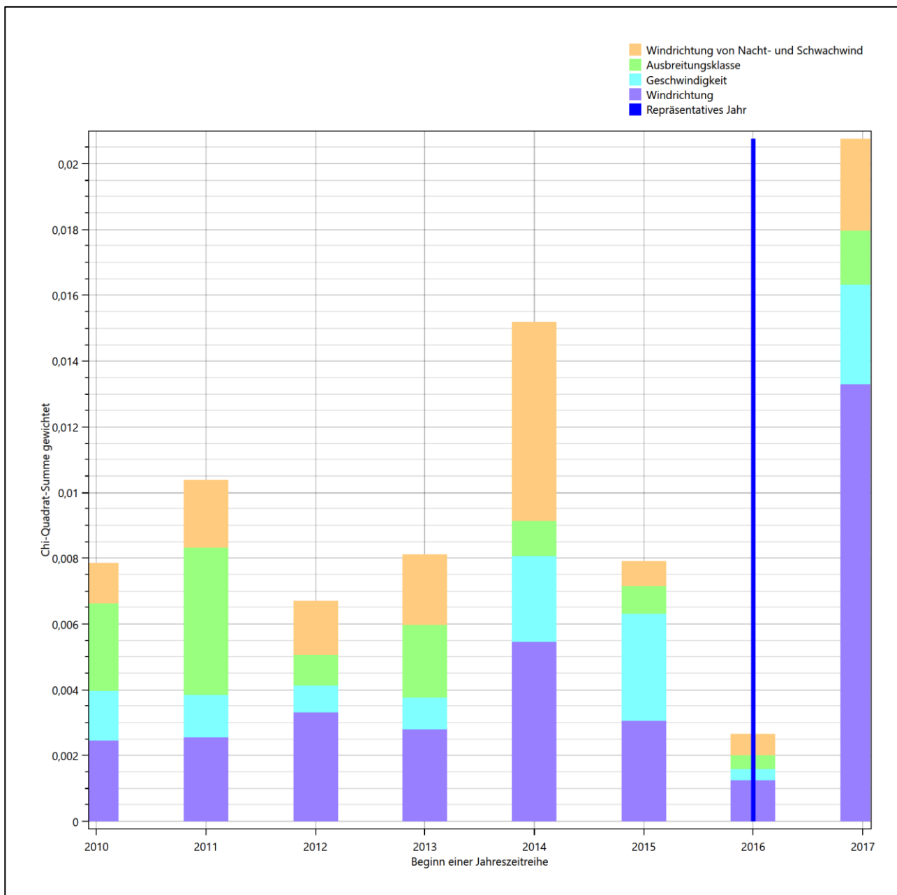
Abbildung 15: Gewichtete \chi^2 -Summe und Einzelwerte als Maß für die Ähnlichkeit der einzelnen Testzeiträume zu je einem Jahr (Jahreszeitreihe) mit dem Gesamtzeitraum
