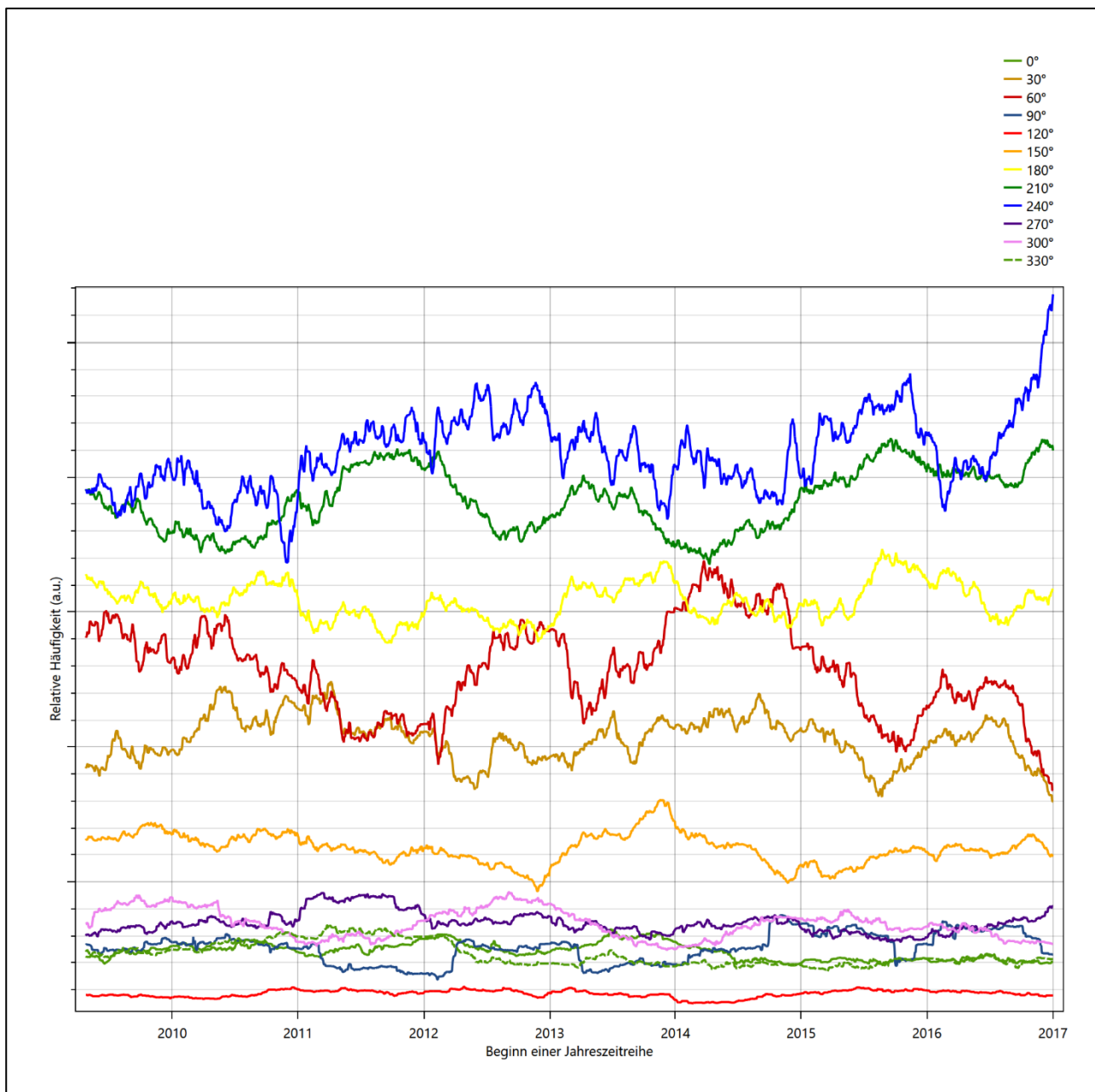
Abbildung 12: Prüfung auf vollständige und homogene Daten der modellierten Daten anhand der Windrichtungsverteilung
