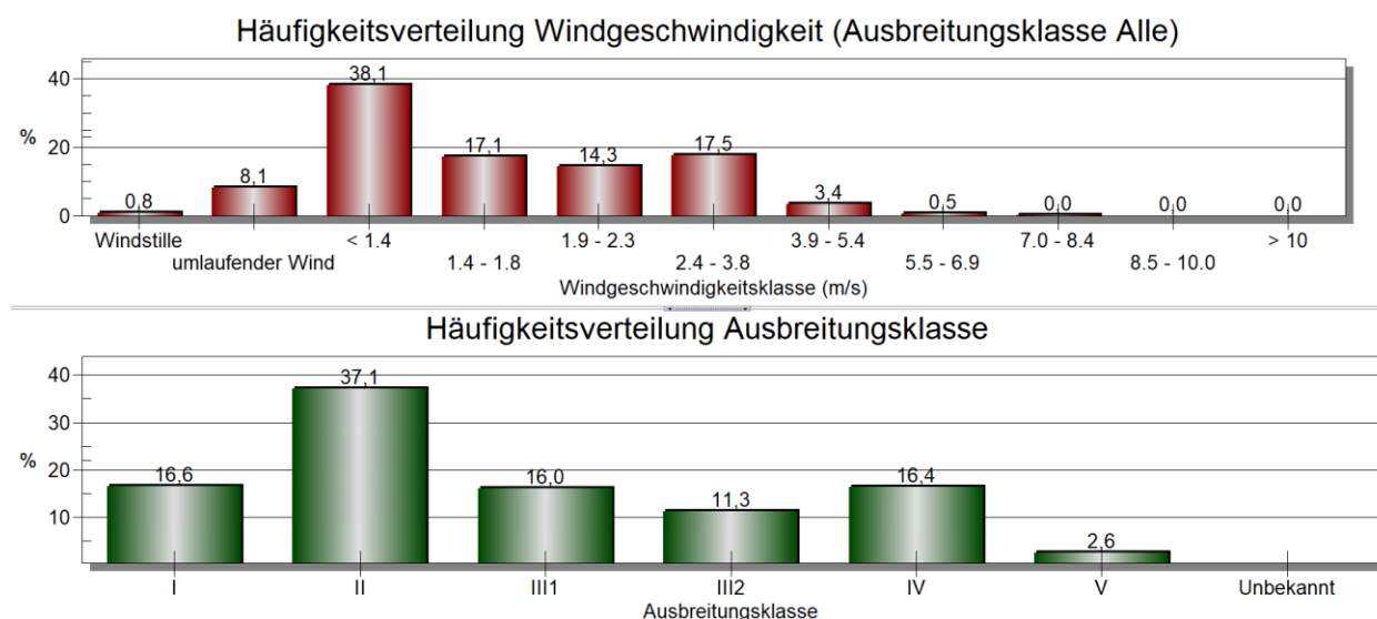
Abbildung 8: Häufigkeitsverteilung der Windgeschwindigkeiten und Ausbreitungsklassen des verwendeten meteorologischen Datensatzes (synAkterm)
