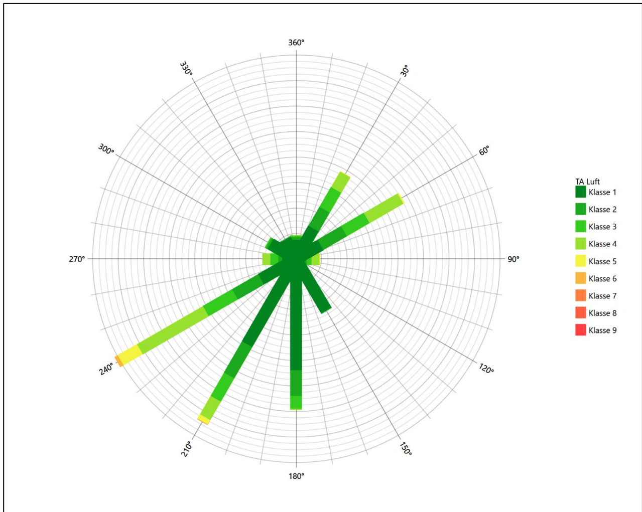
Abbildung 10: Windrichtungsverteilung der modellierten Daten
