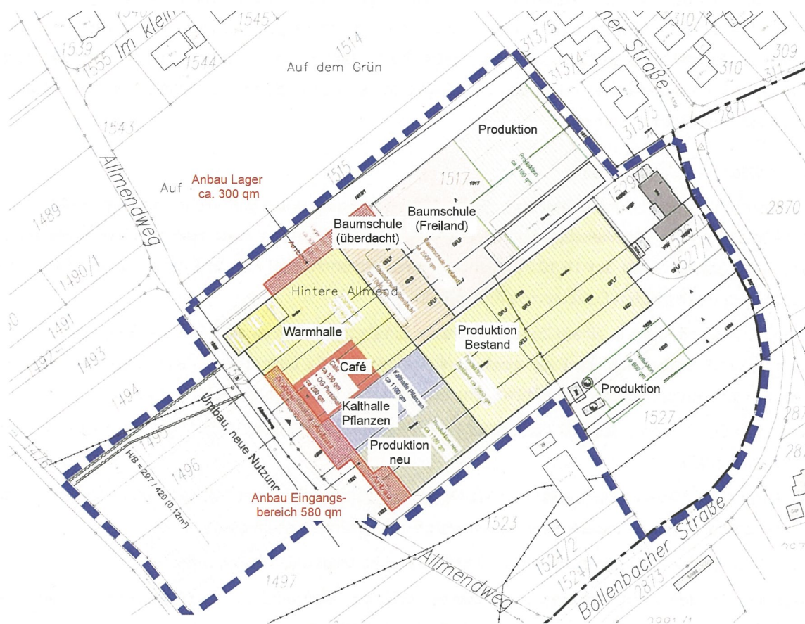
Abb. V-1: Städtebauliche Konzeption
