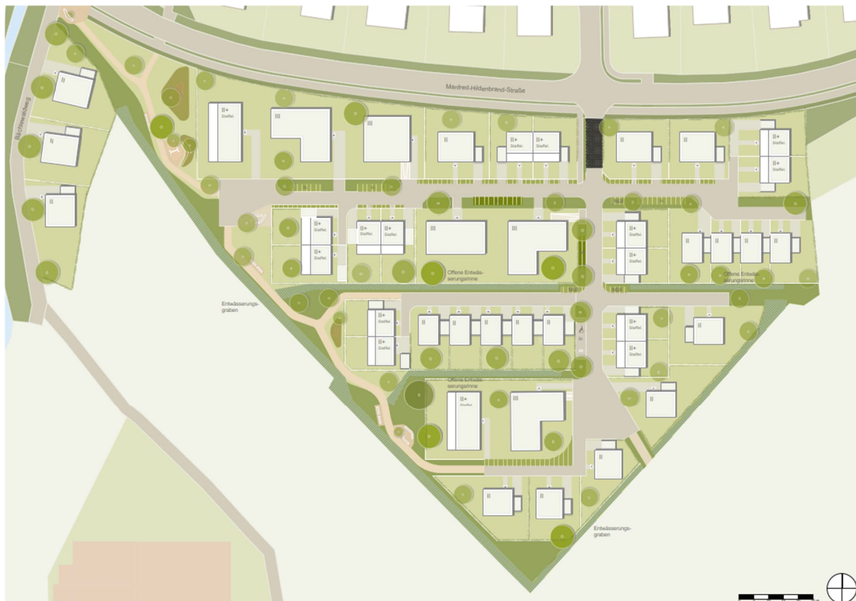
Abb. 1: Städtebaulicher Entwurf. Dachaufsicht / Lageplan. Quelle: (BHM, 2026)
